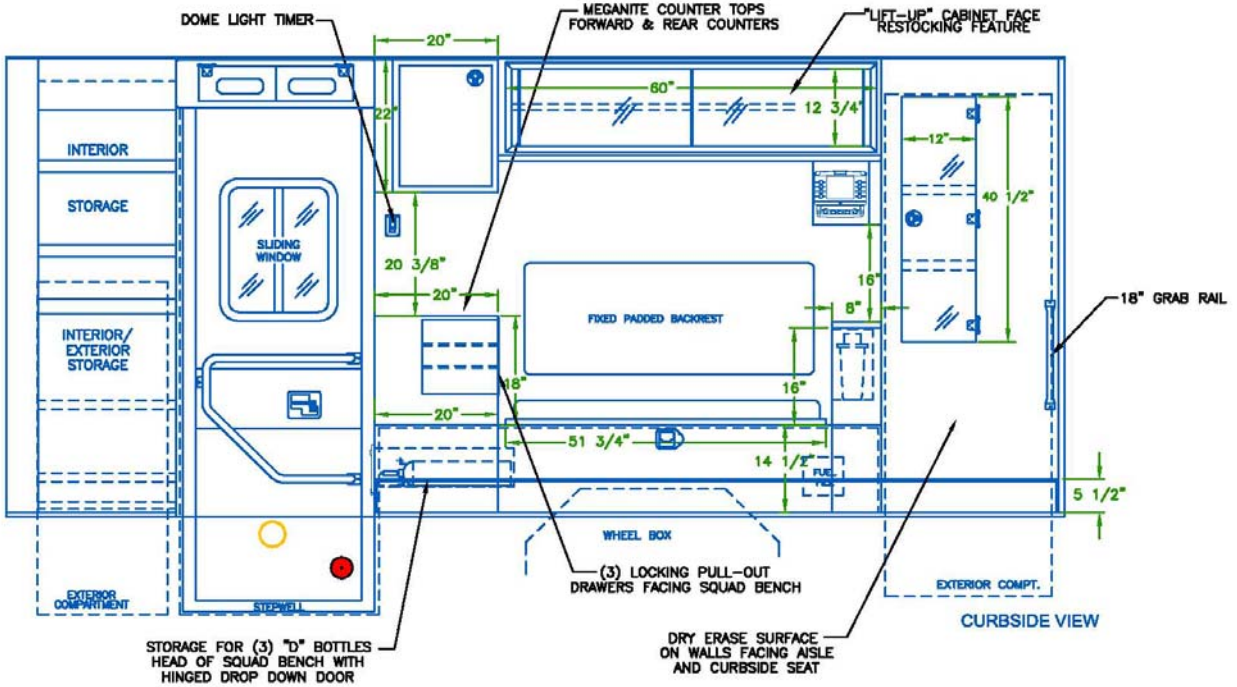
Curbside Layout
