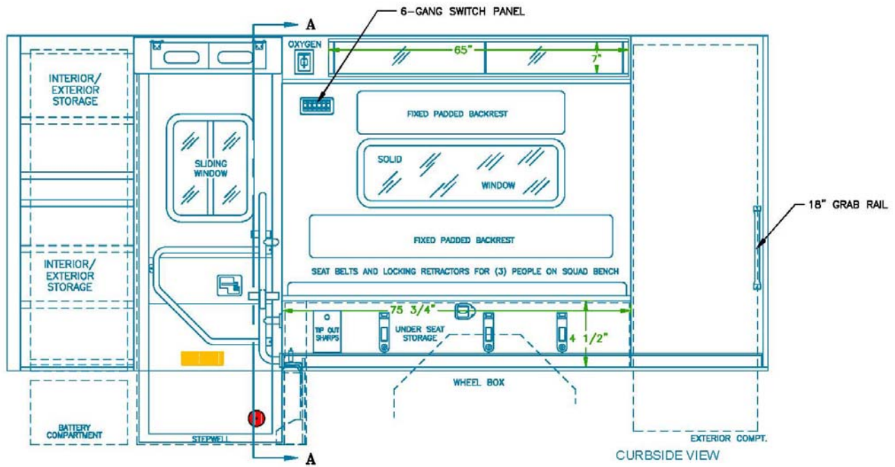
Curbside Layout
