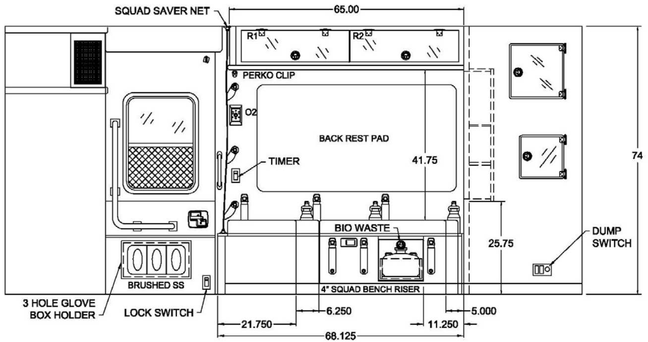
Curbside Layout
